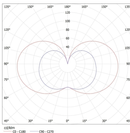
KANLUX S.A. (kat 22660) GIO LED G9-WW / Krzywa rozsyłu światła (biegunowo)
